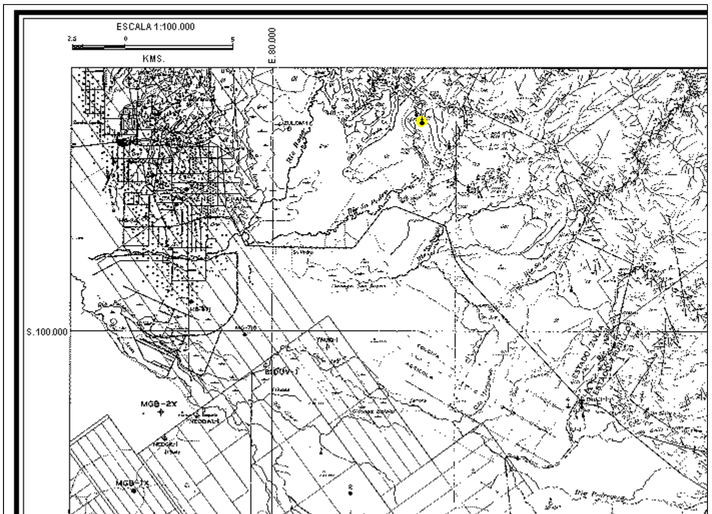
Tomado de: Geología de Superficie de la Creole Petroleum Corporation, Hoja E-4, 1967.
